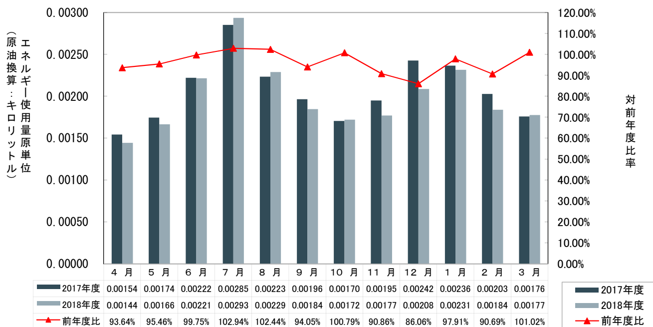
大学全体エネルギー使用量・原単位(原油換算)
