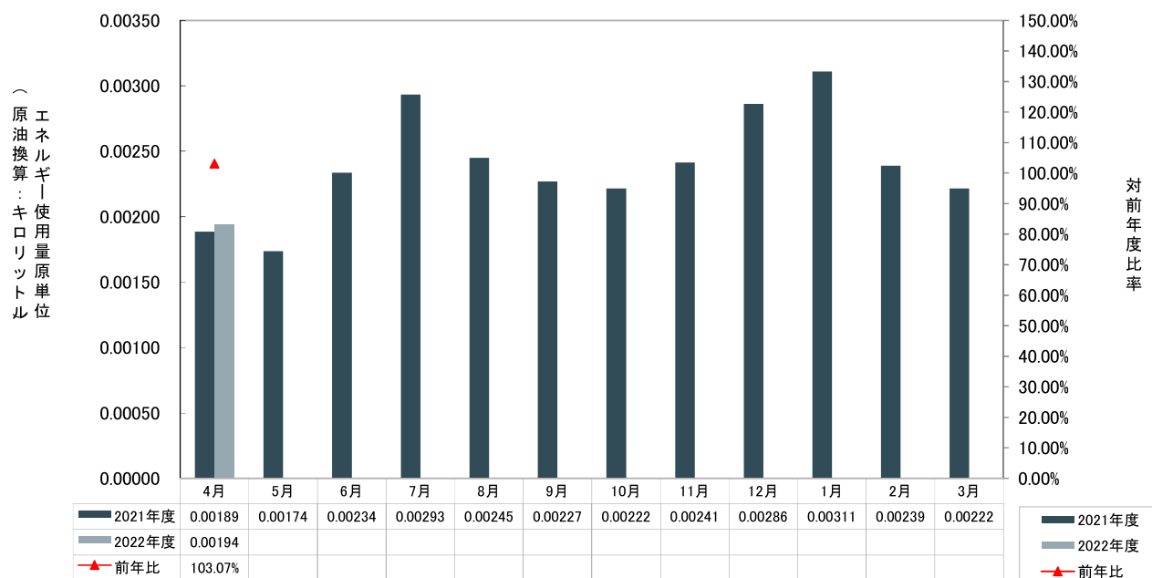
瀬田学舎エネルギー使用量・原単位(原油換算)
