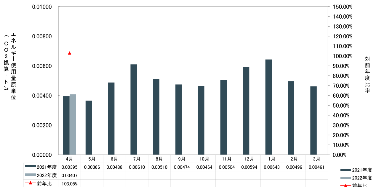
瀬田学舎エネルギー使用量・原単位(CO2換算)
