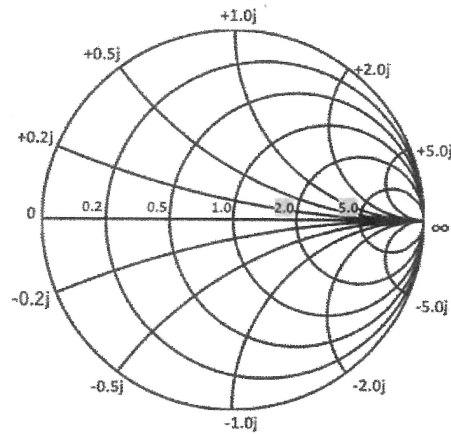
図1 スミスチャート
