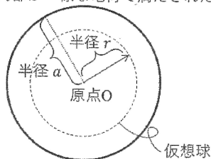
図 1: 球状物質と半径 r の仮想球.
