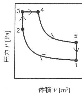
図 1 P - V 線図
