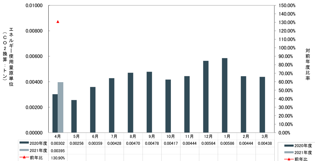
瀬田学舎エネルギー使用量・原単位(CO2換算)
