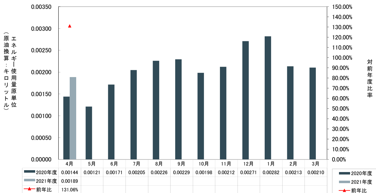
瀬田学舎エネルギー使用量・原単位(原油換算)
